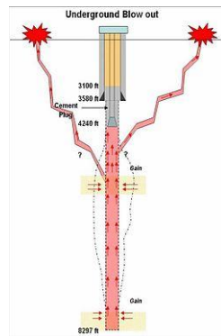
Underground Blowout (semburan liar bawah tanah)
